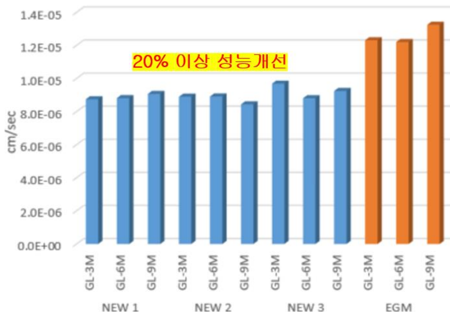
투수시험 결과(평균)
